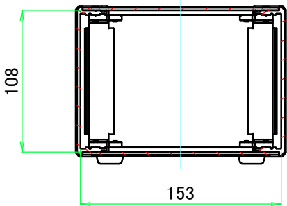
B-B ( 1 : 4 )
