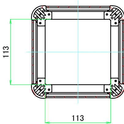
C-C ( 1 : 4 )
